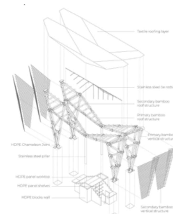
Fig.5 Esploso assonometrico modulo strutturale
